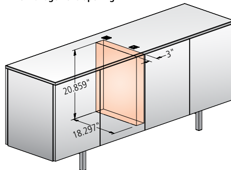
Access Door
