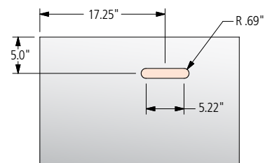
Cutout Dimensions
