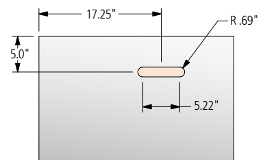
Cutout Dimensions
